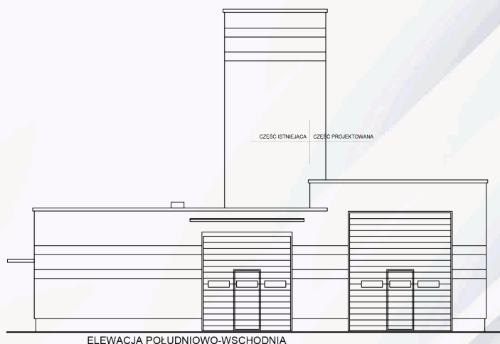
ELEWACJA POŁUDNIOWO-WSCHODNIA
